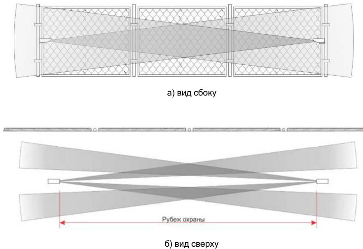
Рисунок 2.2 - Двухнаправленная схема установки извещателей
